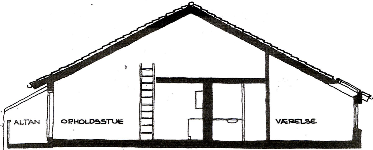
SNIT I TAGLEJLIGHED VED OVENLYSVINDUE
